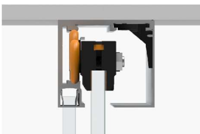
TECHO CON VIDRIO FIJO
